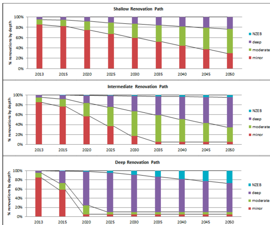
Fig. 13. Scenarii de renovare superficială, intermediară și aprofundată
